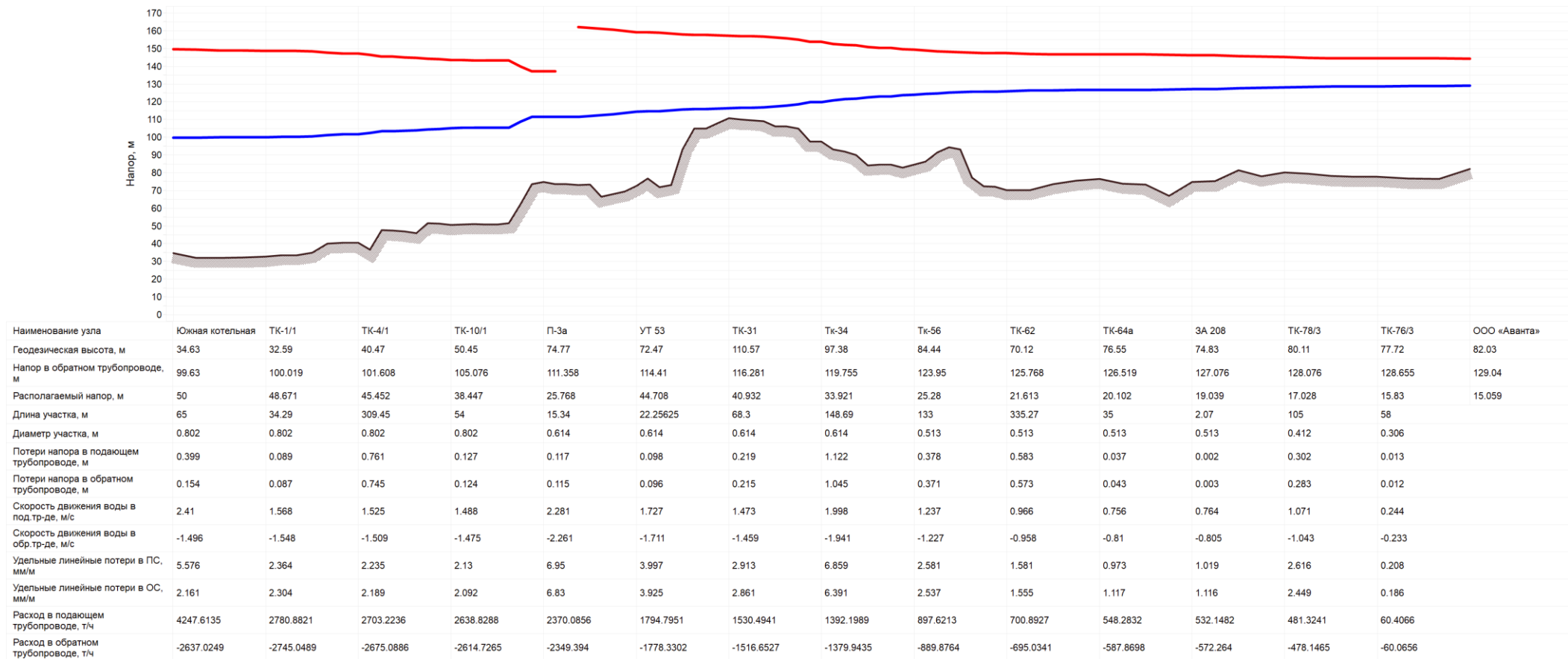
Рисунок 4.8 Пьезометрический график участка тепловой сети от Южной котельной до ООО «Аванта»
