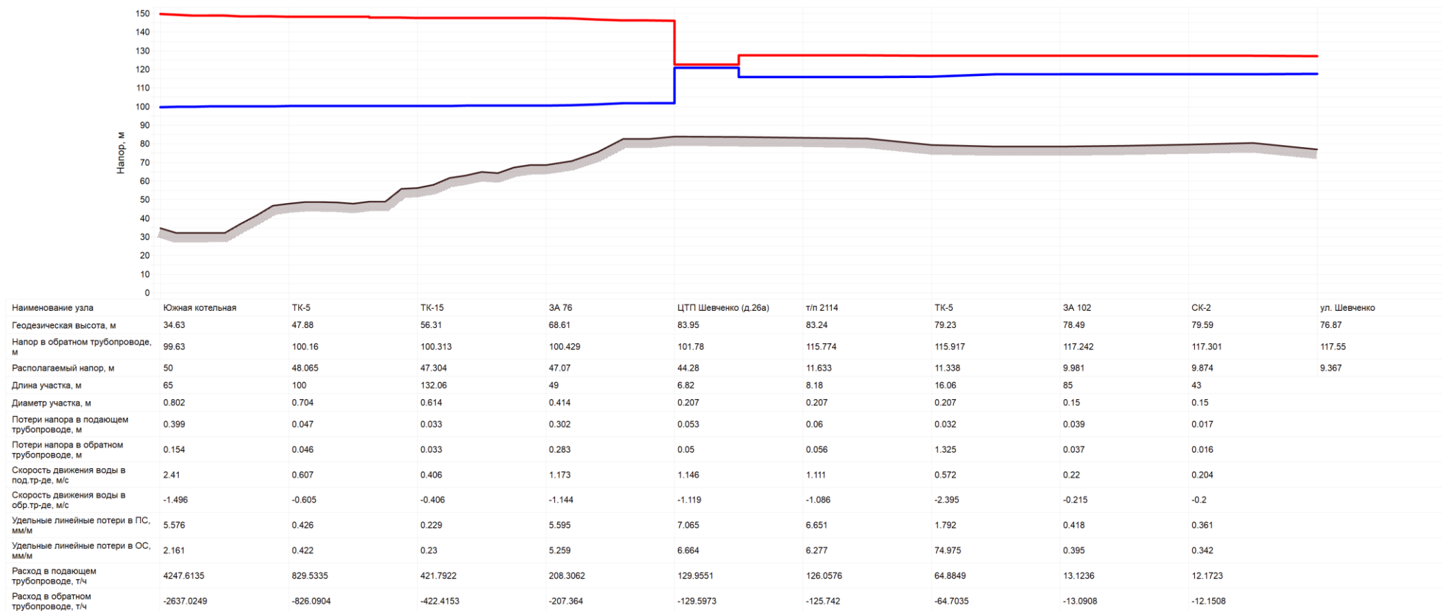
Рисунок 4.10 Пьезометрический график участка тепловой сети от Южной котельной до перспективного потребителя ул. Шевченко
