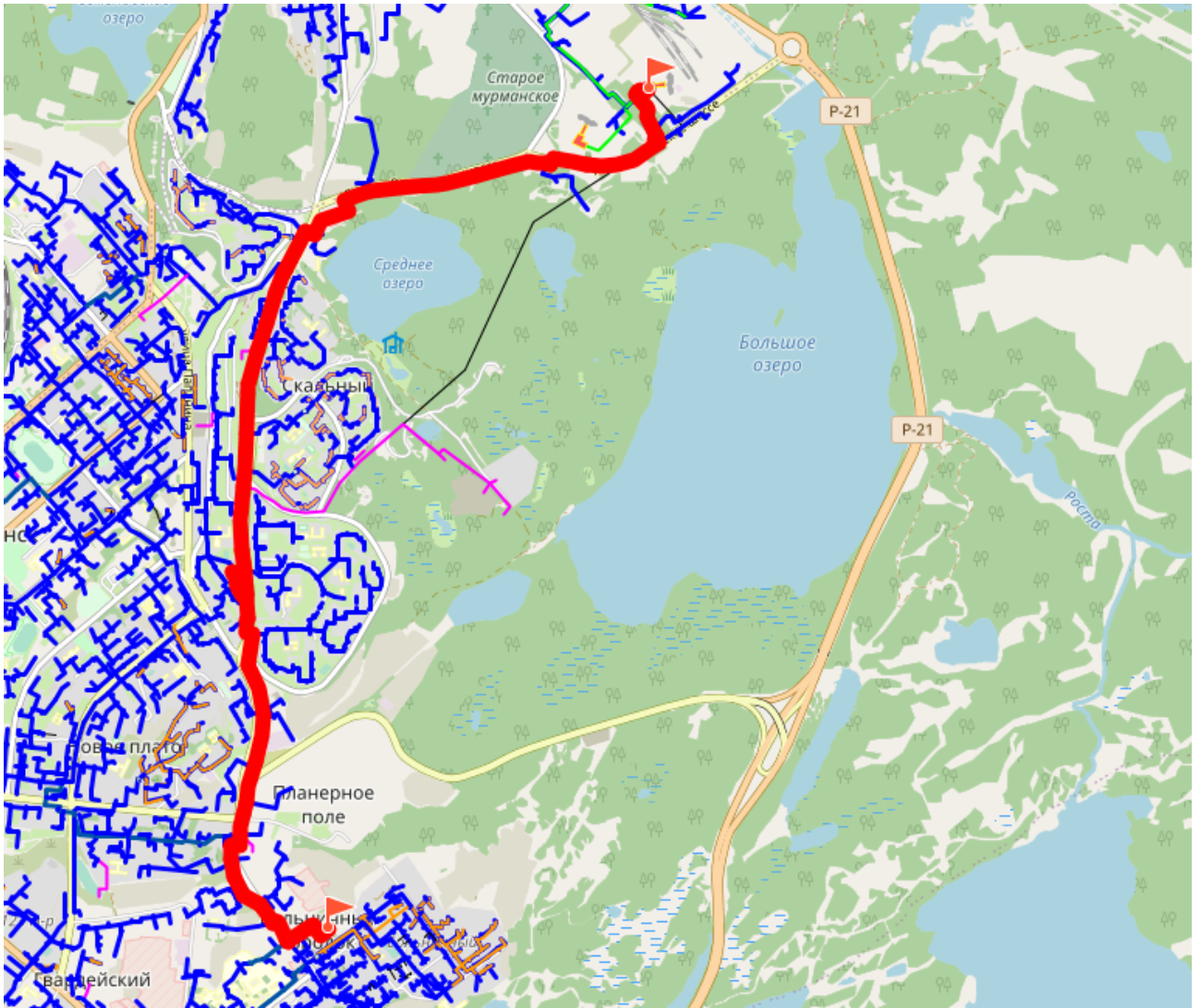
Рисунок 4.15 Путь для построения пьезометрического графика от Восточной котельной до застройки в Больничном городке
