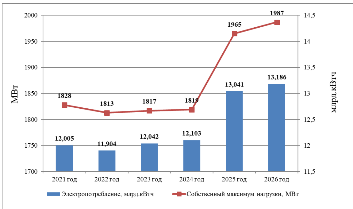
Рисунок 7.4 Уровни потребления электроэнергии и мощности на территории Мурманской области на 2021-2026 годы. Базовый вариант.
