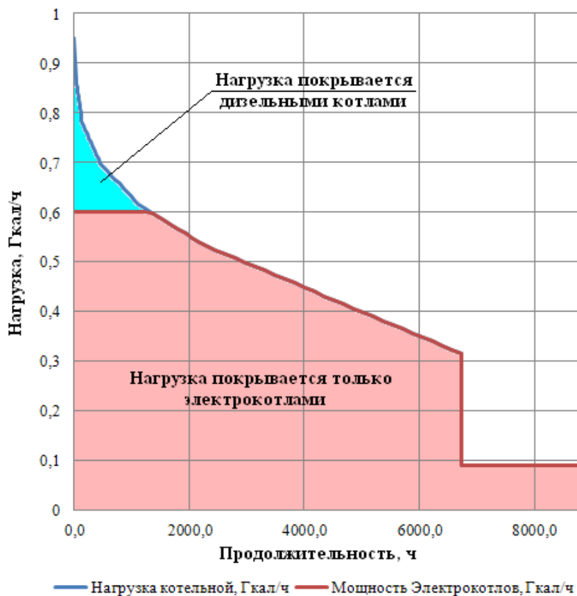
Рисунок 7.10 График Россандера при работе электрокотлов
