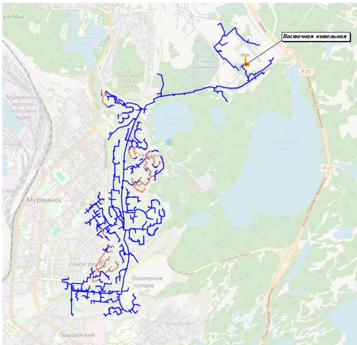
Рисунок 11.34. Схема тепловых сетей от Восточной котельной
