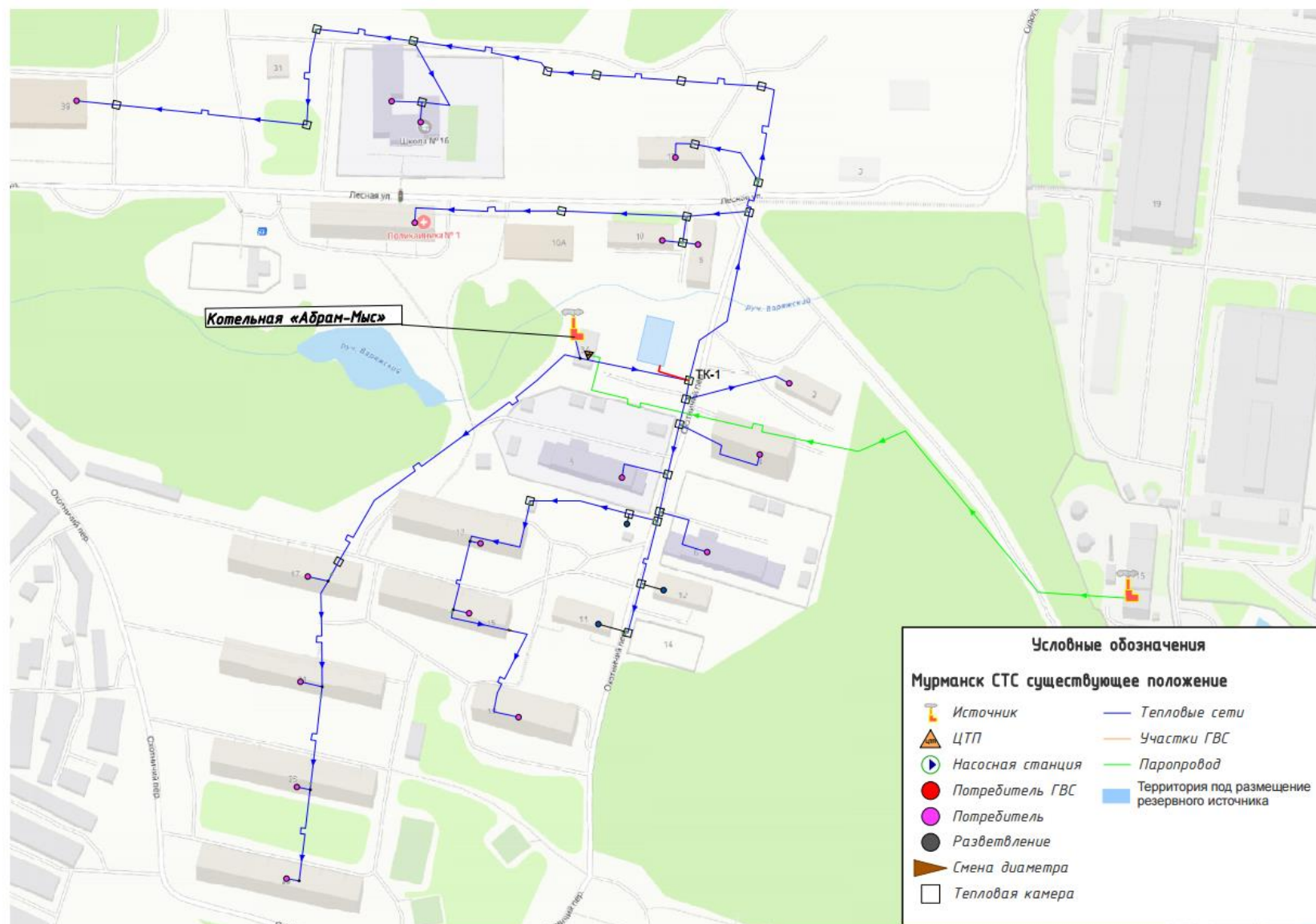
Рисунок 11.28. Места размещения передвижной котельной установки и точки подключения к сетям теплоснабжения в случае возникновения аварийной ситуации на источнике тепловой энергии жилого района Абрам-Мыс
