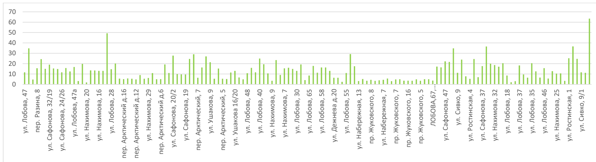
Рисунок 11.16. Средний суммарный недоотпуск теплоты потребителям котельной «Роста»
