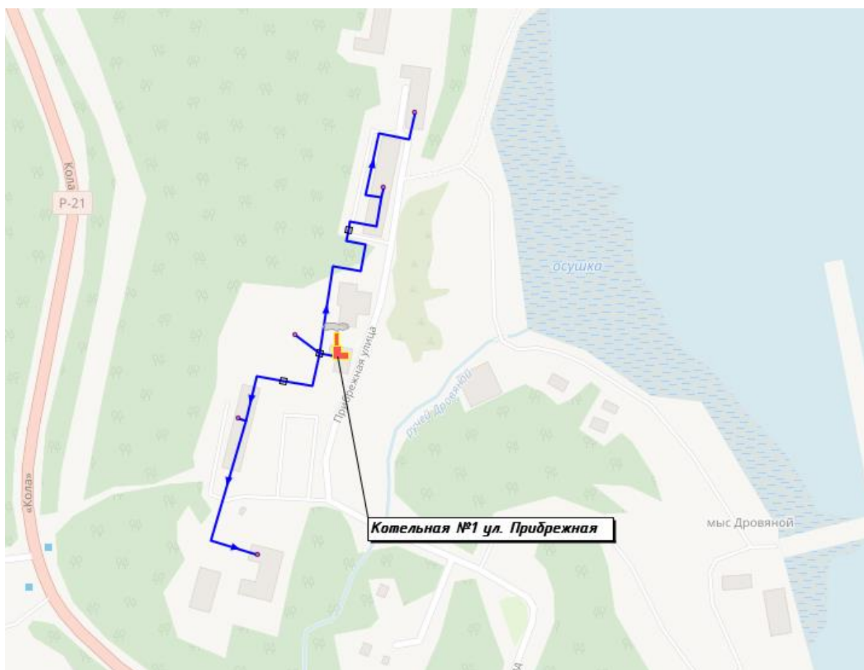
Рисунок 11.46. Схема тепловых сетей от котельной №1 ул. Прибрежная
