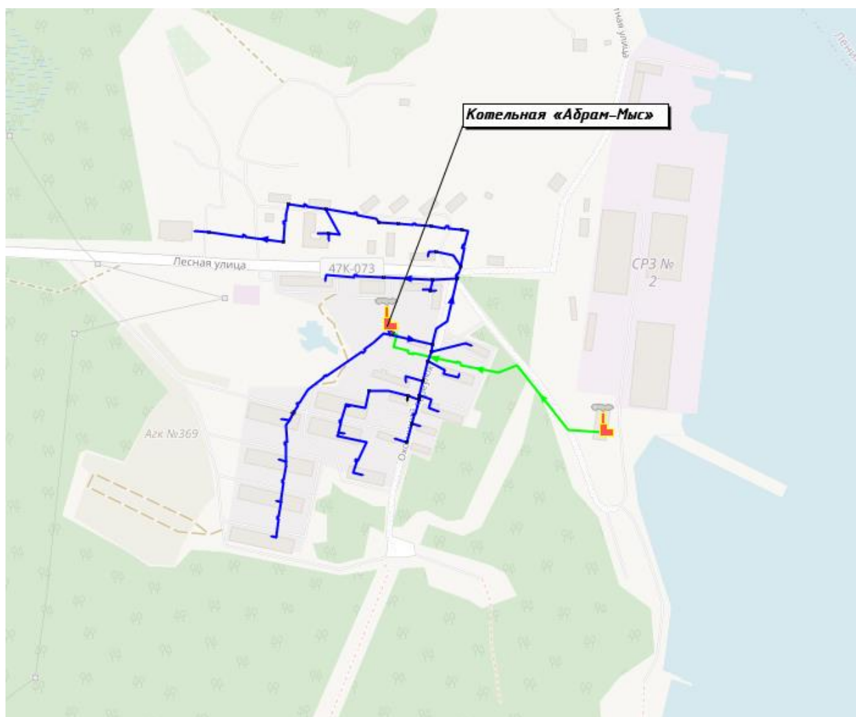
Рисунок 11.43. Схема тепловых сетей от котельной «Абрам-Мыс»
