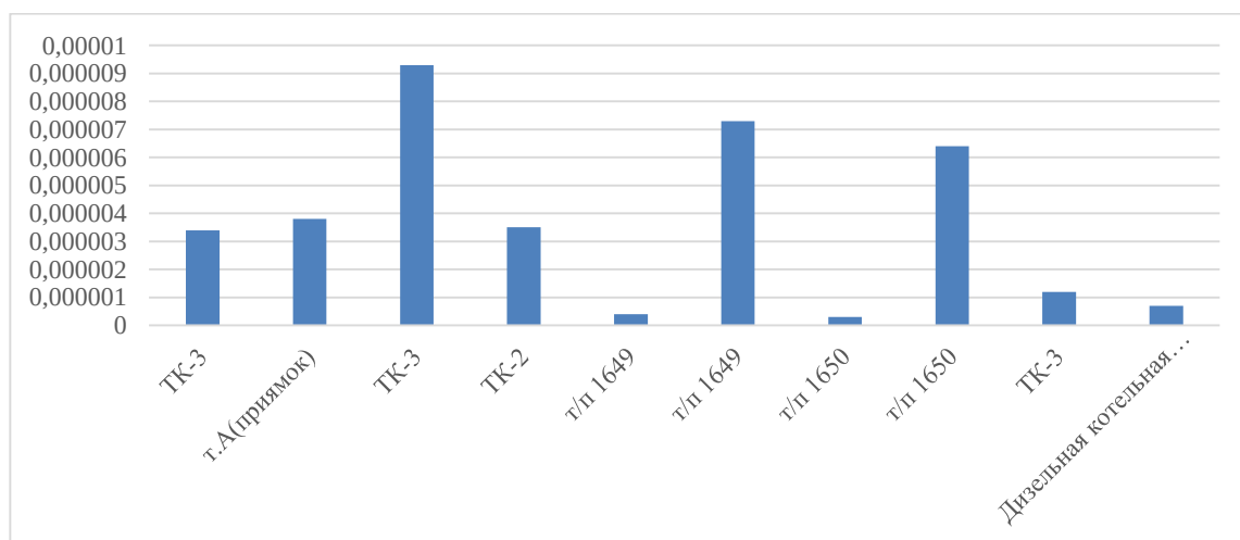
Рисунок 11.2. Вероятность отказа работоспособного состояния тепловой сети от котельной №1 ул.Прибрежная
