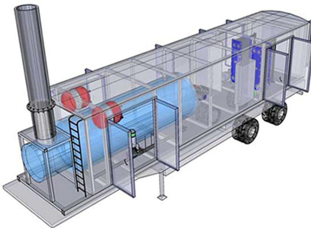
Рисунок 11.27. Схематичный вид передвижной котельной установки
