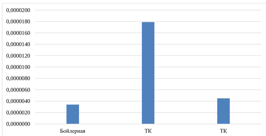
Рисунок 11.13.Верятность отказа работоспособного состояния тепловой сети от котельной № 22
