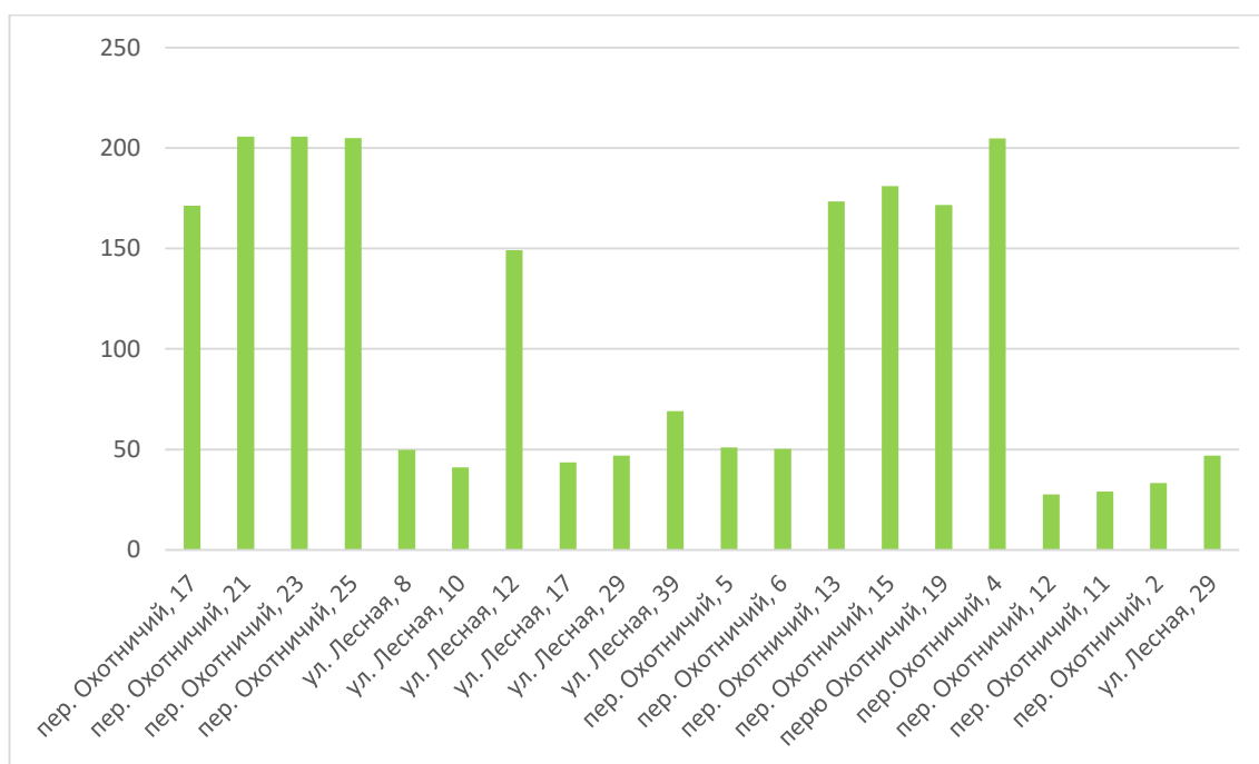
Рисунок 11.14. Средний суммарный недоотпуск теплоты потребителям котельной «Абрам-Мыс»
