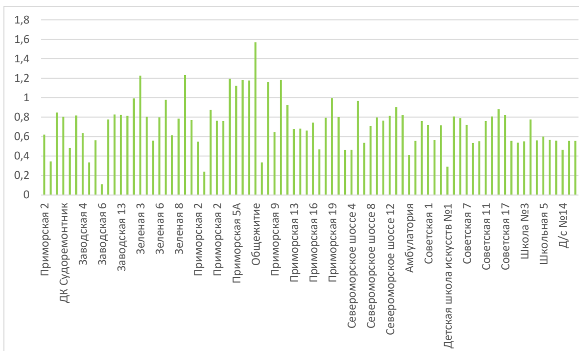
Рисунок 11.23. Средний суммарный недоотпуск теплоты потребителям котельной ТЦ «Росляково-1»
