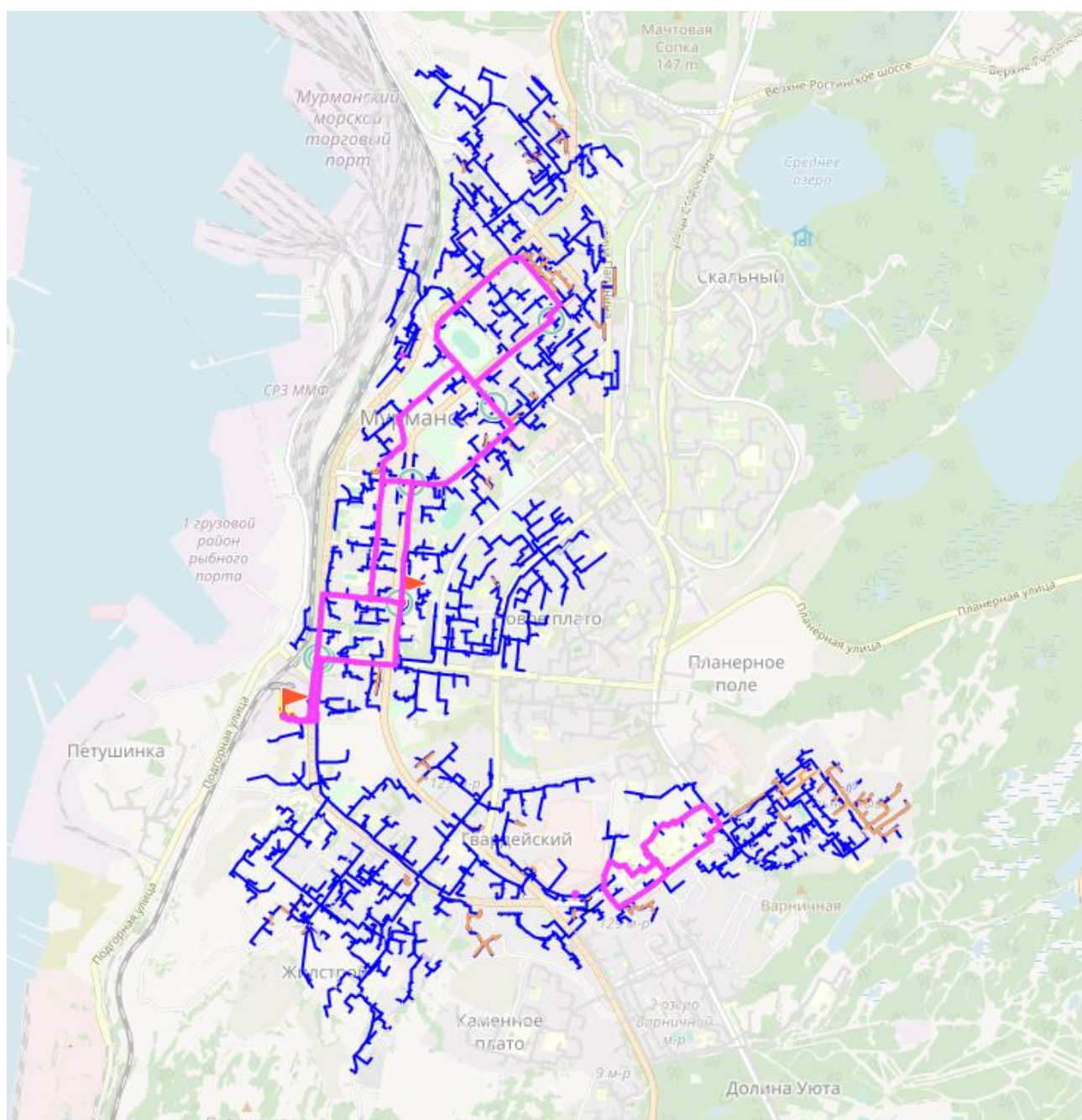
Рисунок 11.36. Моделировании аварийной ситуации на тепловых сетях от Мурманской ТЭЦ
