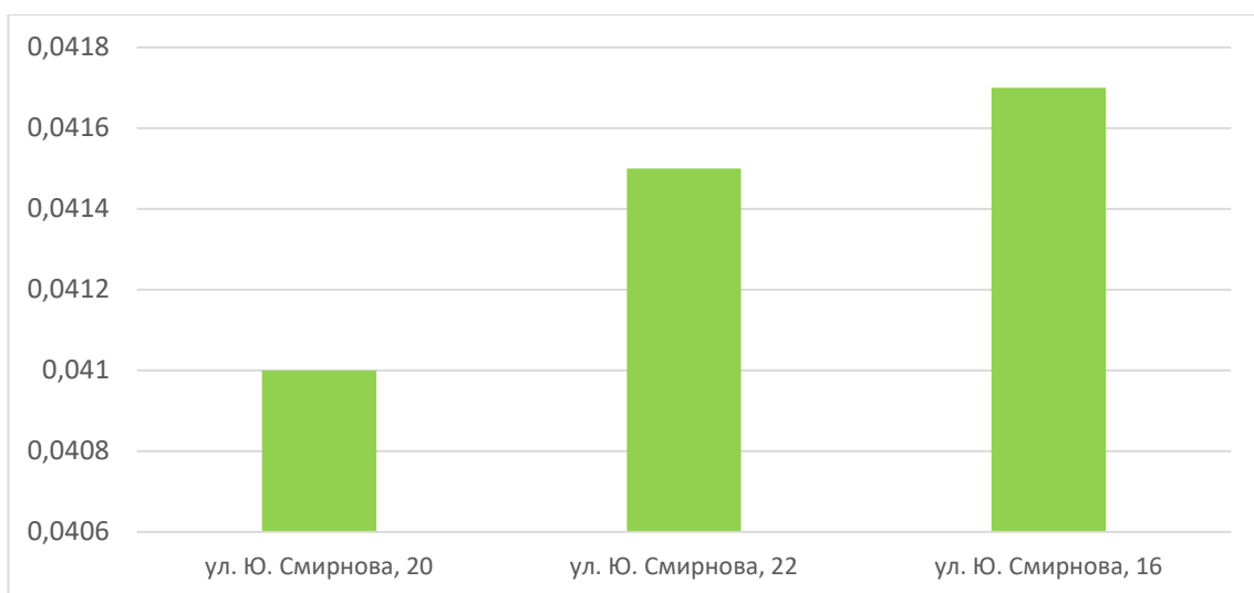
Рисунок 11.20. Средний суммарный недоотпуск теплоты потребителям угольной котельной
