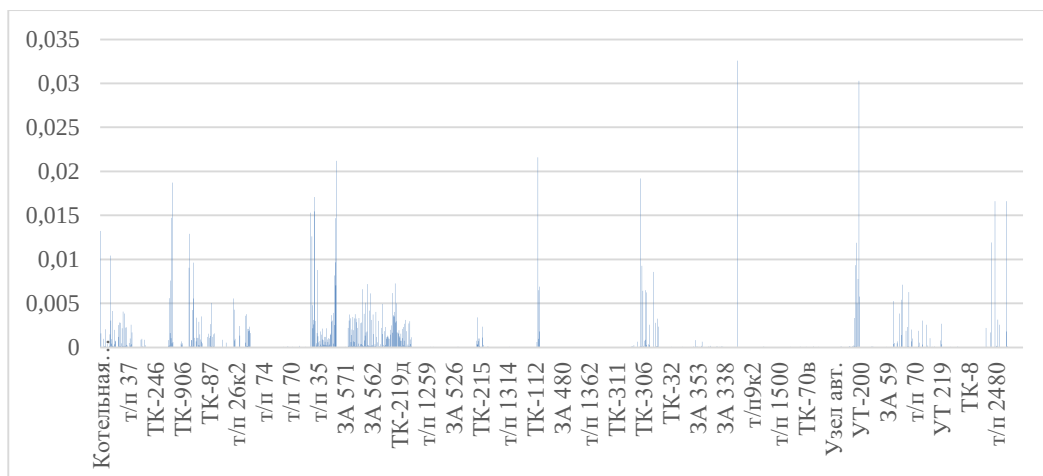
Рисунок 11.6. Вероятность отказа работоспособного состояния тепловой сети от котельной АО «ММТП»
