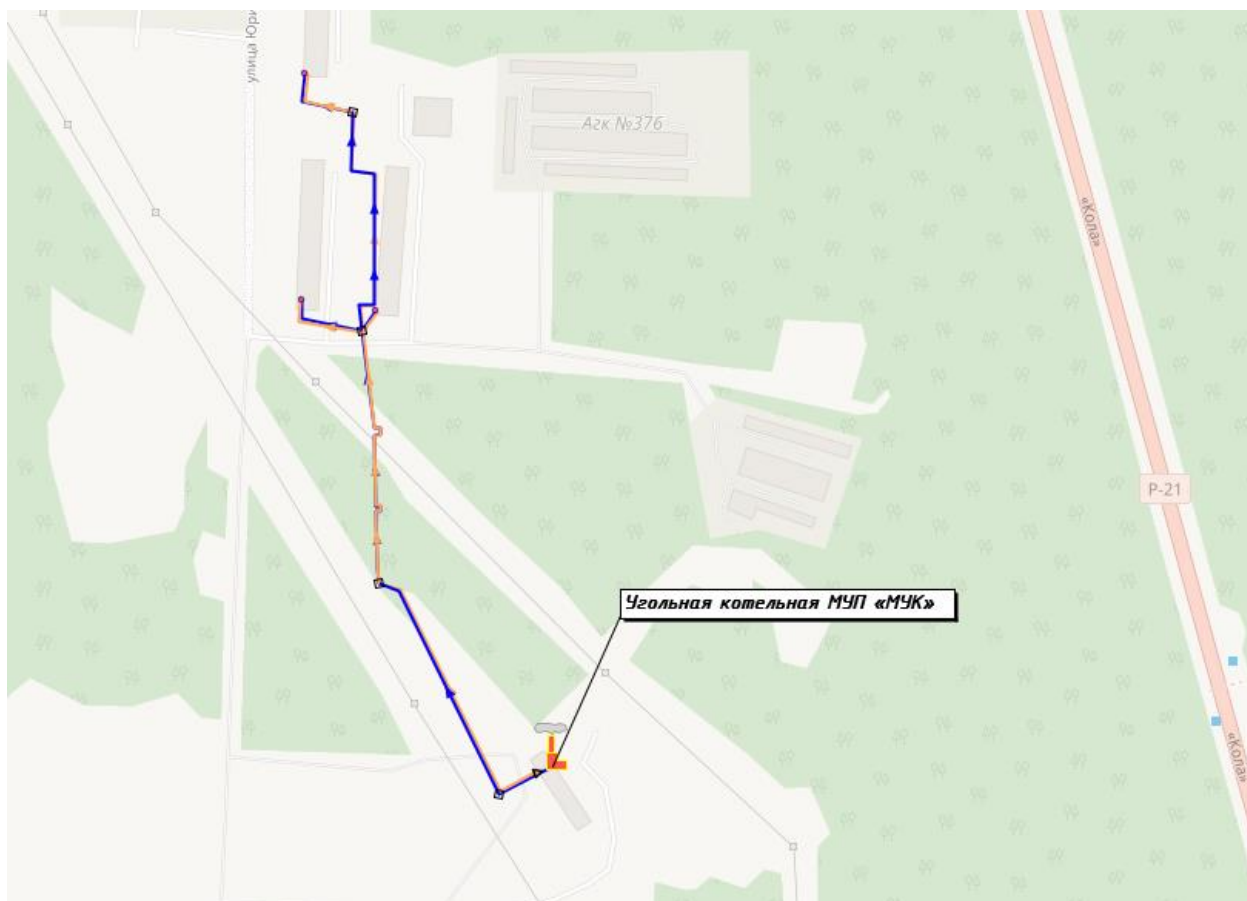
Рисунок 11.48. Схема тепловых сетей от угольной котельной
