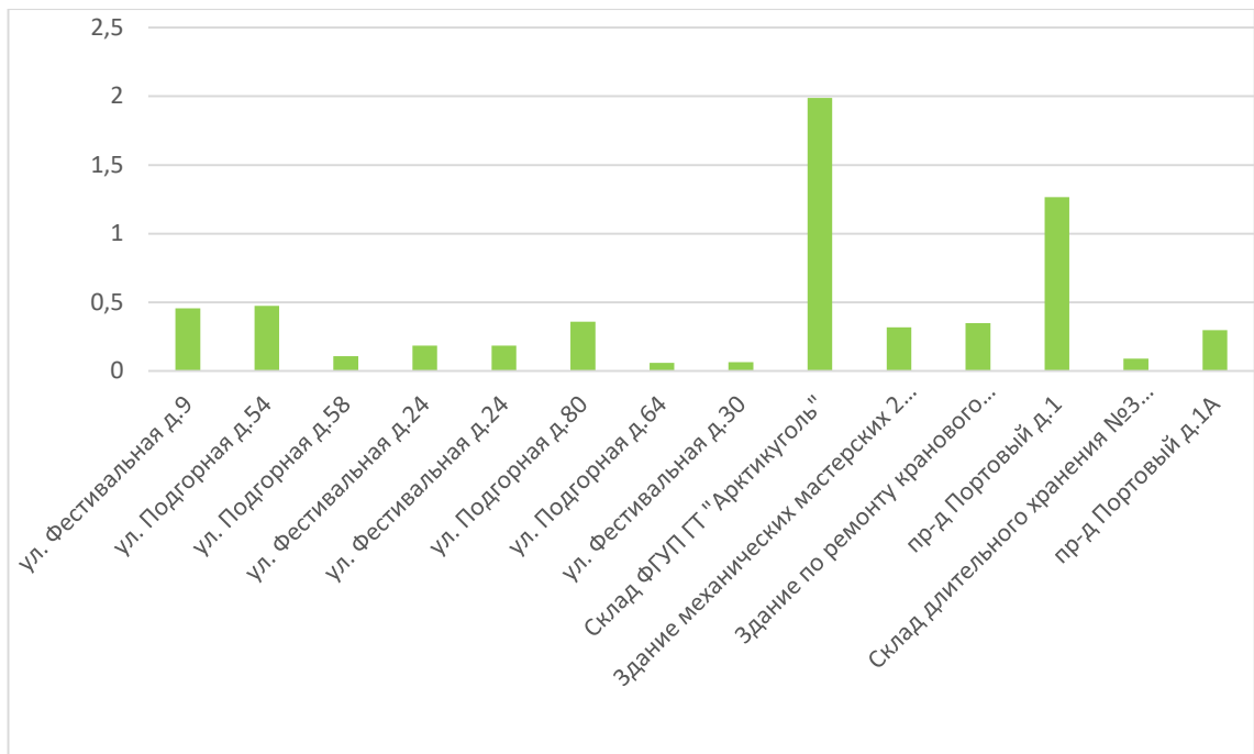
Рисунок 11.18.Средний суммарный недоотпуск теплоты потребителям котельной «Фестивальная»
