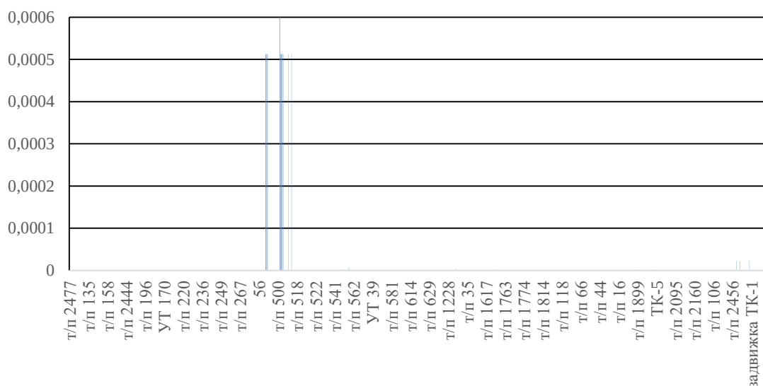
Рисунок 11.1. Вероятность отказа работоспособного состояния тепловой сети от Восточной котельной
