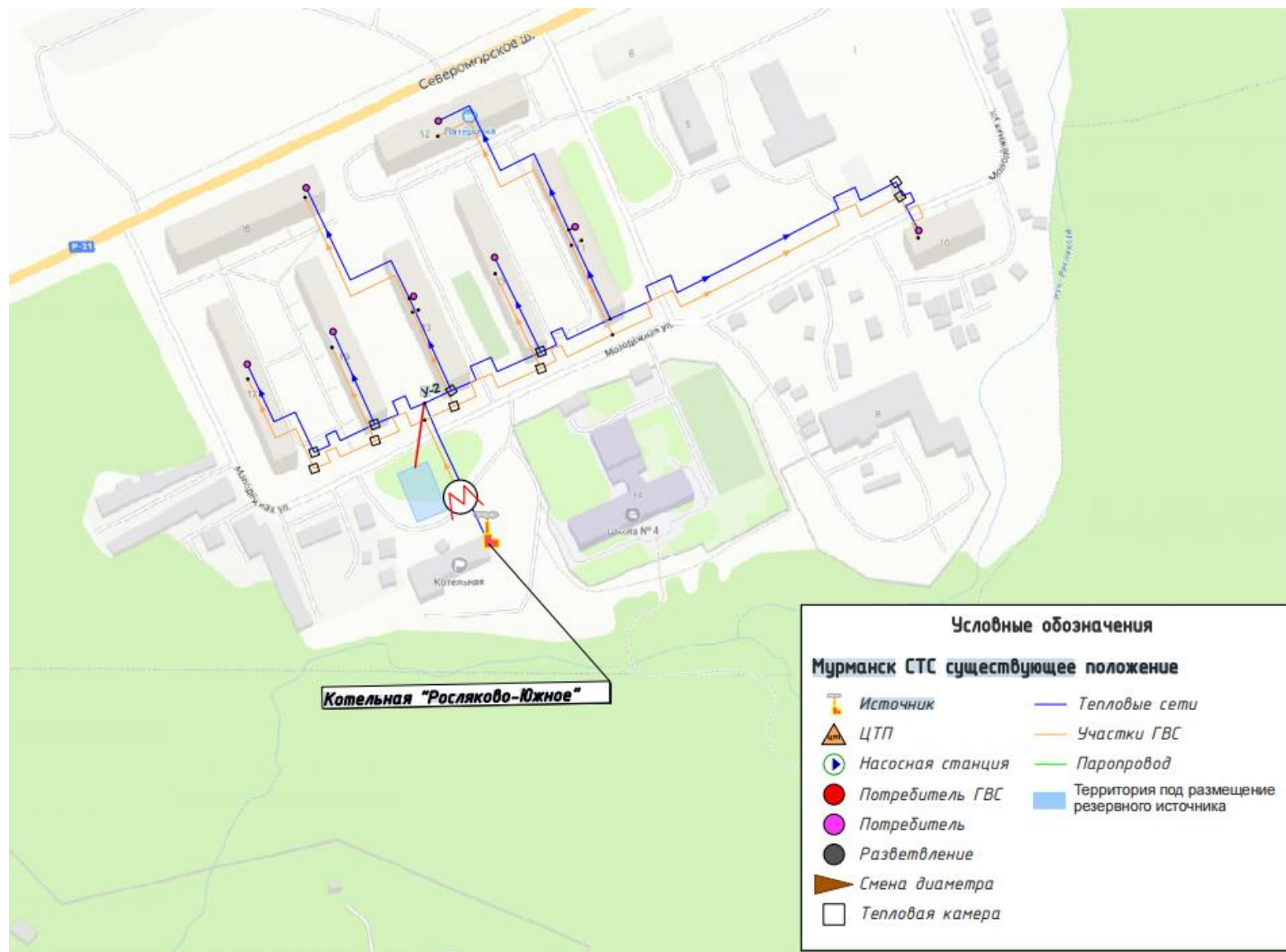
Рисунок 11.30. Место размещения передвижной котельной установки и точки подключения к сетям теплоснабжения в случае возникновения аварийной ситуации на источнике тепловой энергии жилого района Росляково (Малое Росляково)
