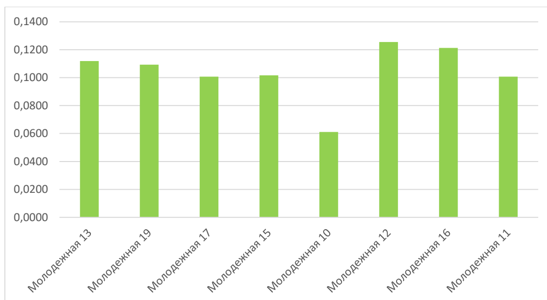
Рисунок 11.24. Средний суммарный недоотпуск теплоты потребителям котельной «Росляково-Южное»
