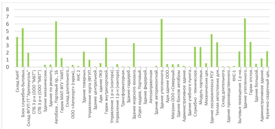
Рисунок 11.22. Средний суммарный недоотпуск теплоты потребителям котельной АО «ММТП»
