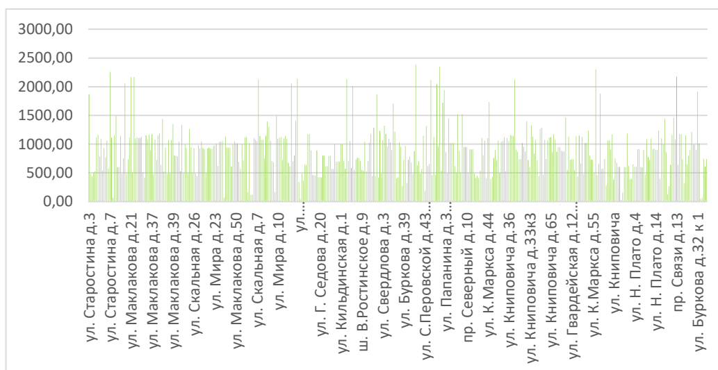
Рисунок 11.25. Средний суммарный недоотпуск теплоты потребителям Восточной котельной
