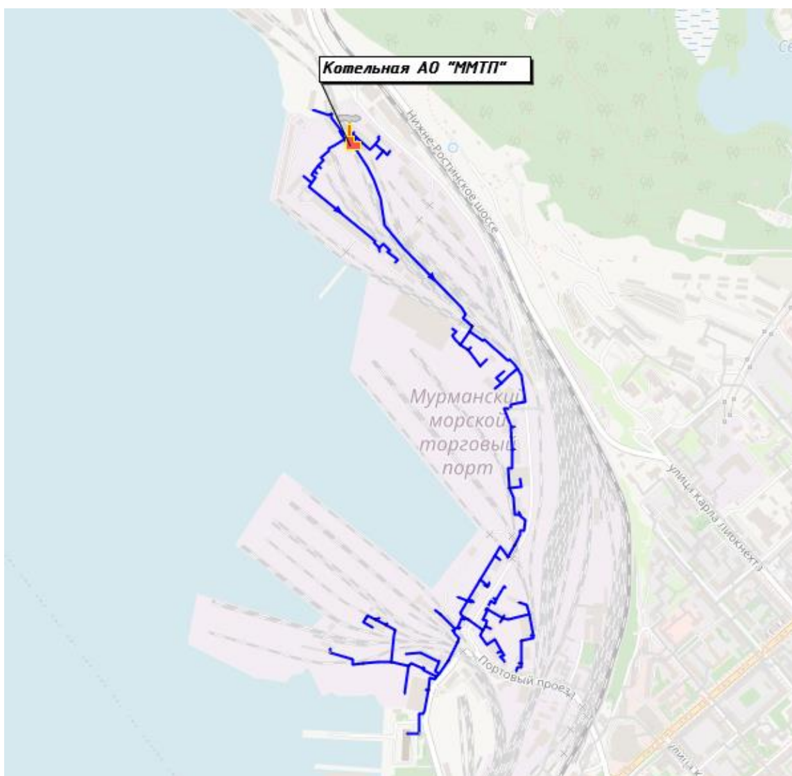
Рисунок 11.47. Схема тепловых сетей от котельной АО «ММТП»
