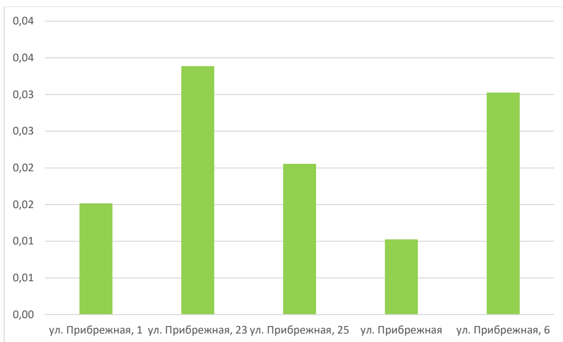
Рисунок 11.15. Средний суммарный недоотпуск теплоты потребителям дизельной котельной ООО «ТЛК»
