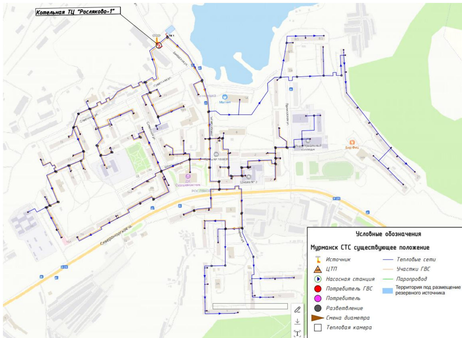
Рисунок 11.29. Места размещения передвижной котельной установки и точки подключения к сетям теплоснабжения в случае возникновения аварийной ситуации на источнике тепловой энергии жилого района Росляково
