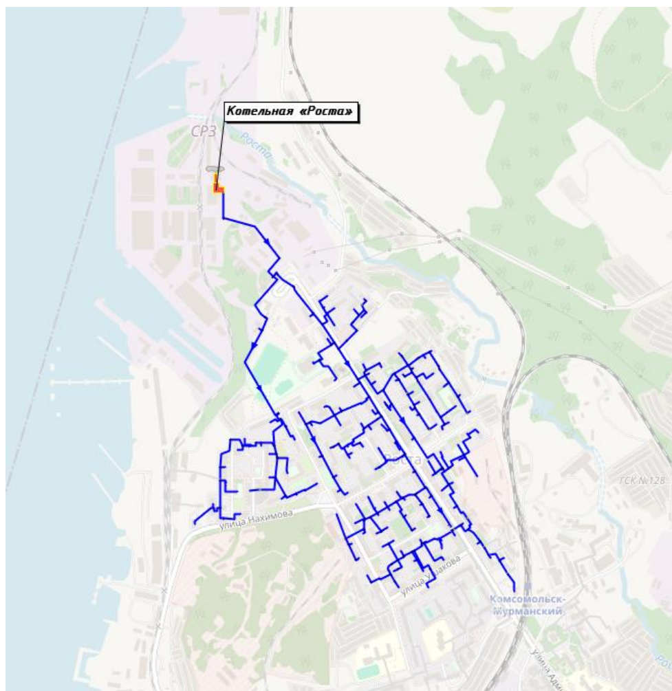
Рисунок 11.41. Схема тепловых сетей от котельной «Роста»
