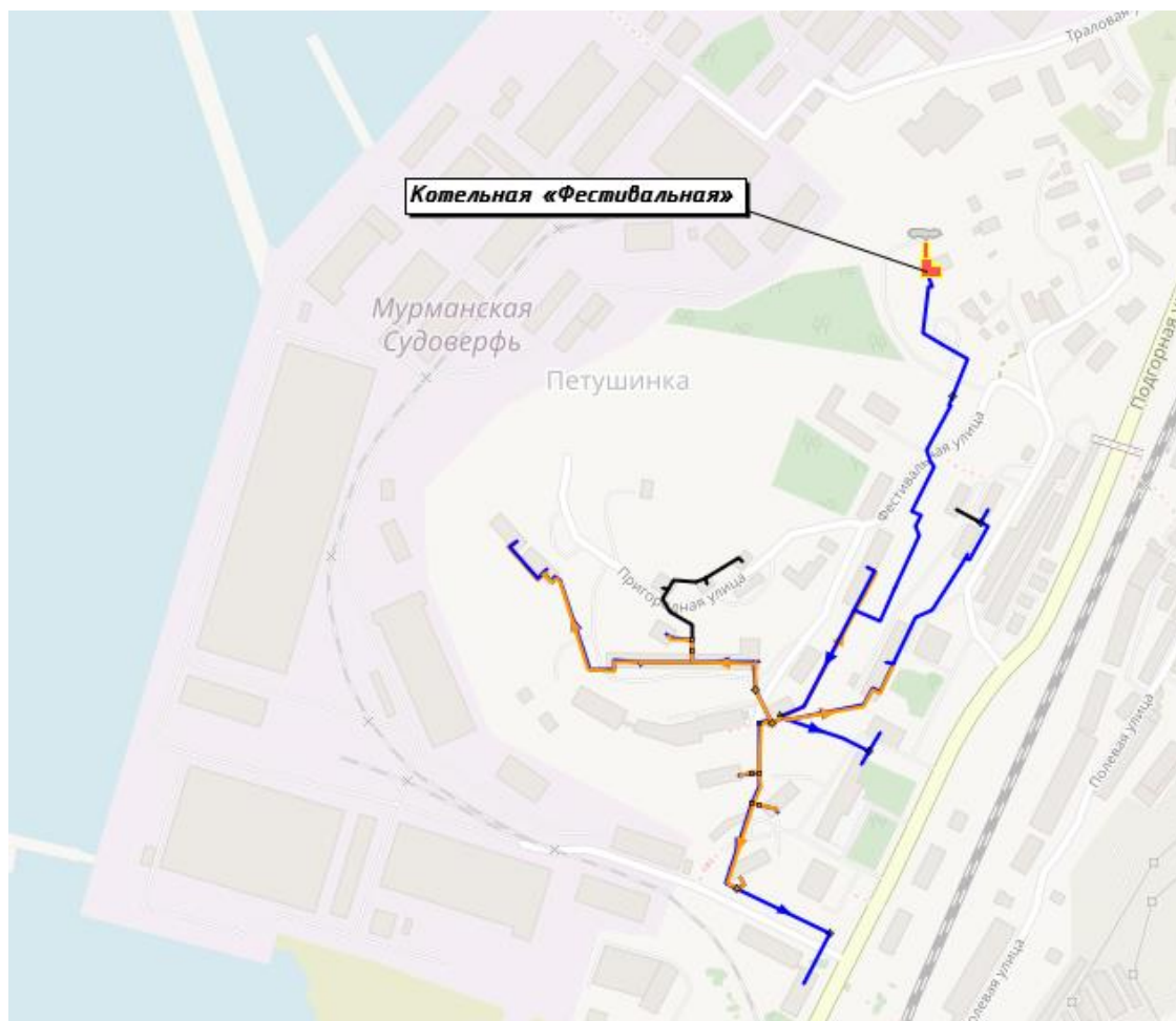
Рисунок 11.44. Схема тепловых сетей от котельной «Абрам-Мыс»
