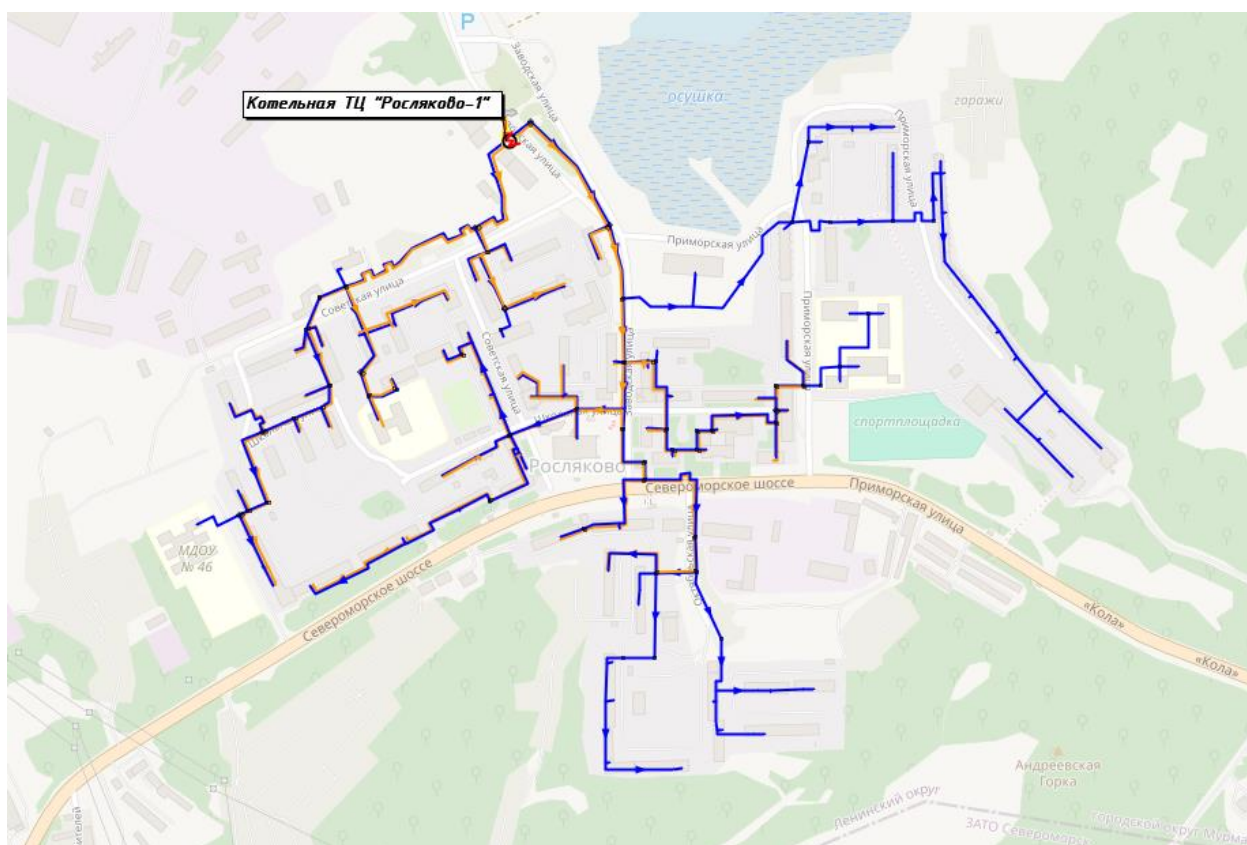
Рисунок 11.45. Схема тепловых сетей от котельной ТЦ «Росляково-1»
