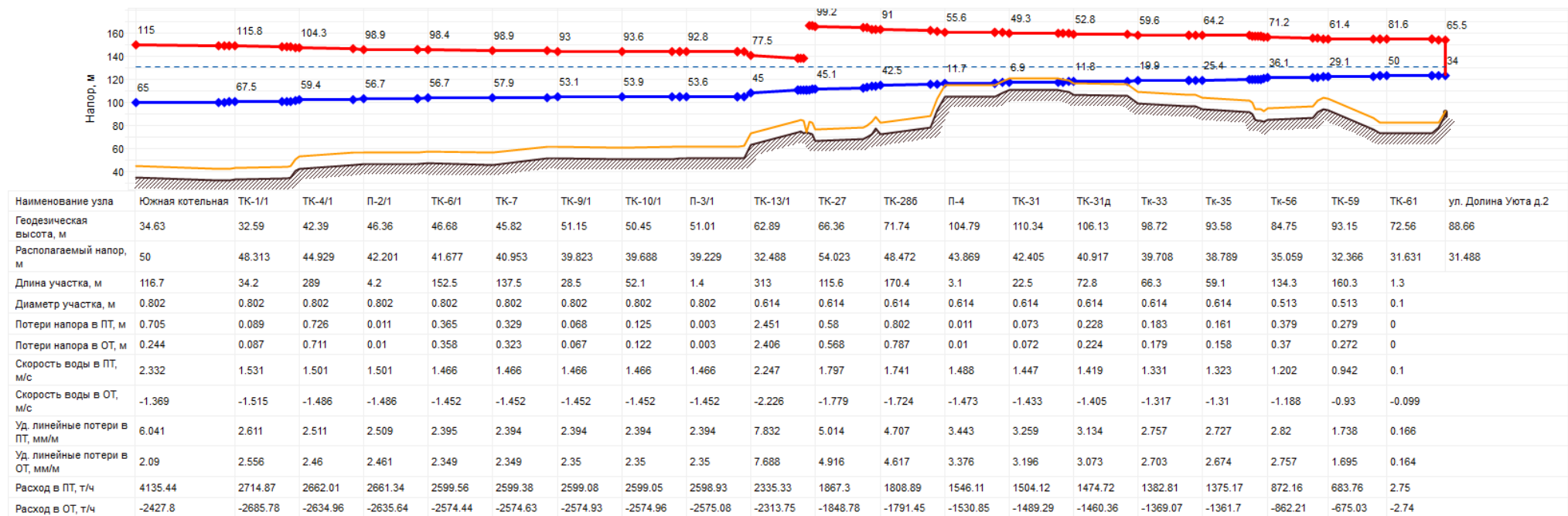
Рисунок 3.29 Существующий гидравлический режим тепловых сетей от Южной котельной
