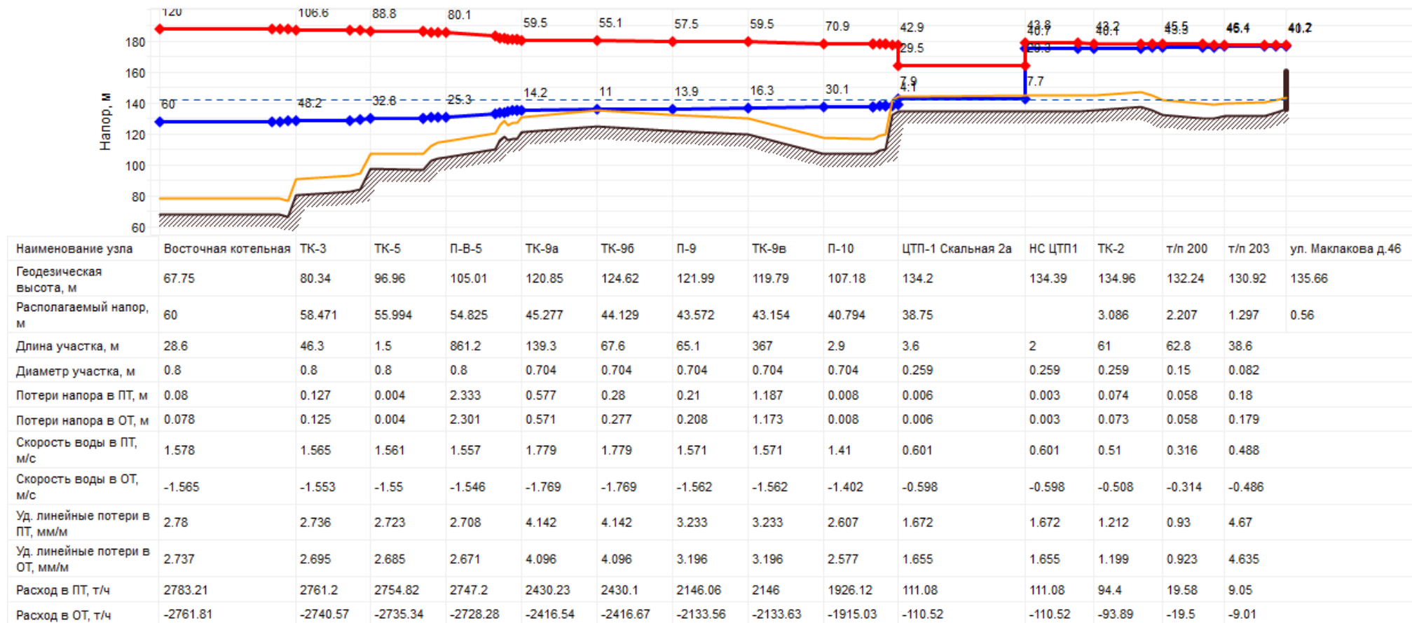
Рисунок 3.28 Существующий гидравлический режим тепловых сетей от Восточной котельной
