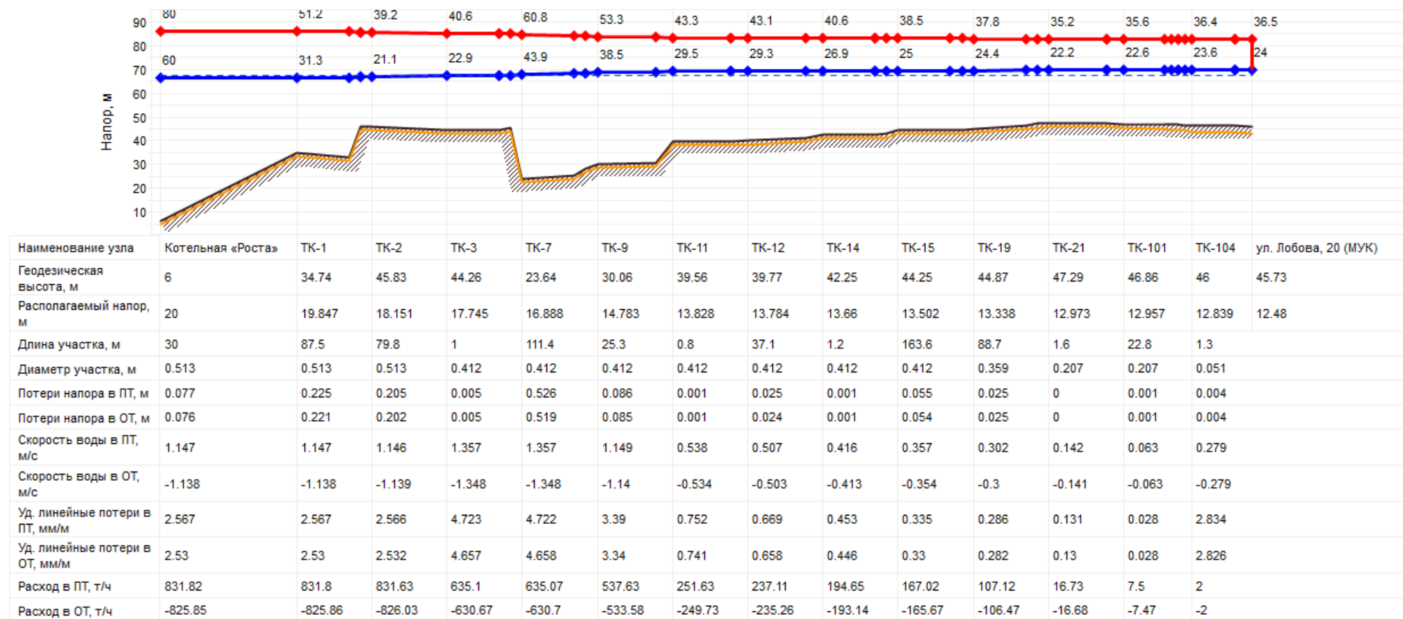
Рисунок 3.31 Существующий гидравлический режим тепловых сетей от котельной «Роста»
