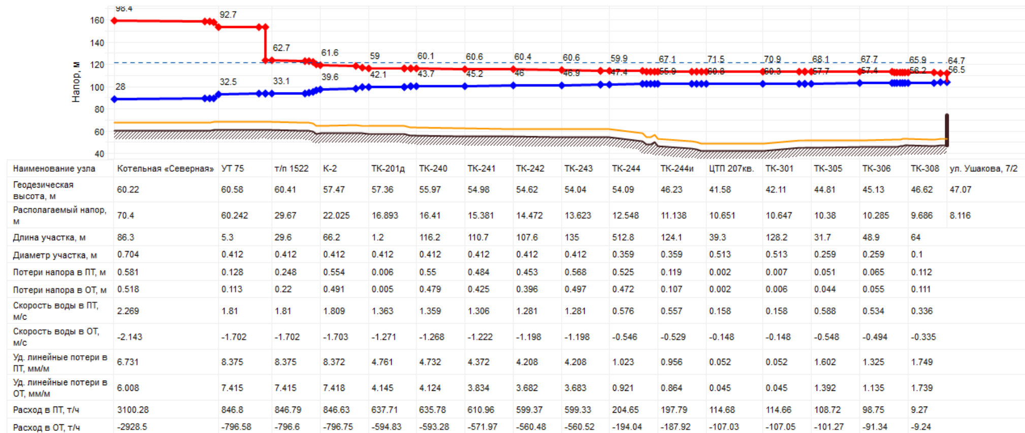
Рисунок 3.30 Существующий гидравлический режим тепловых сетей от Северной котельной
