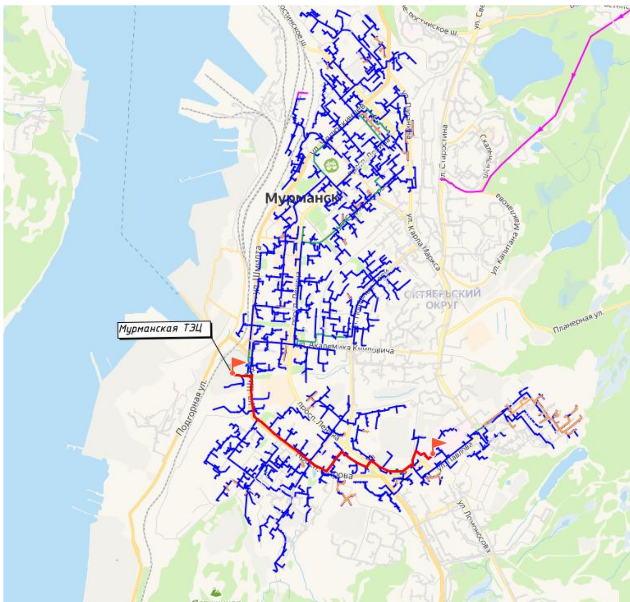
Рисунок 4.7 Путь для построения пьезометрического графика от Мурманской ТЭЦ до потребителя ул.Павлова, д.6, корп.2
