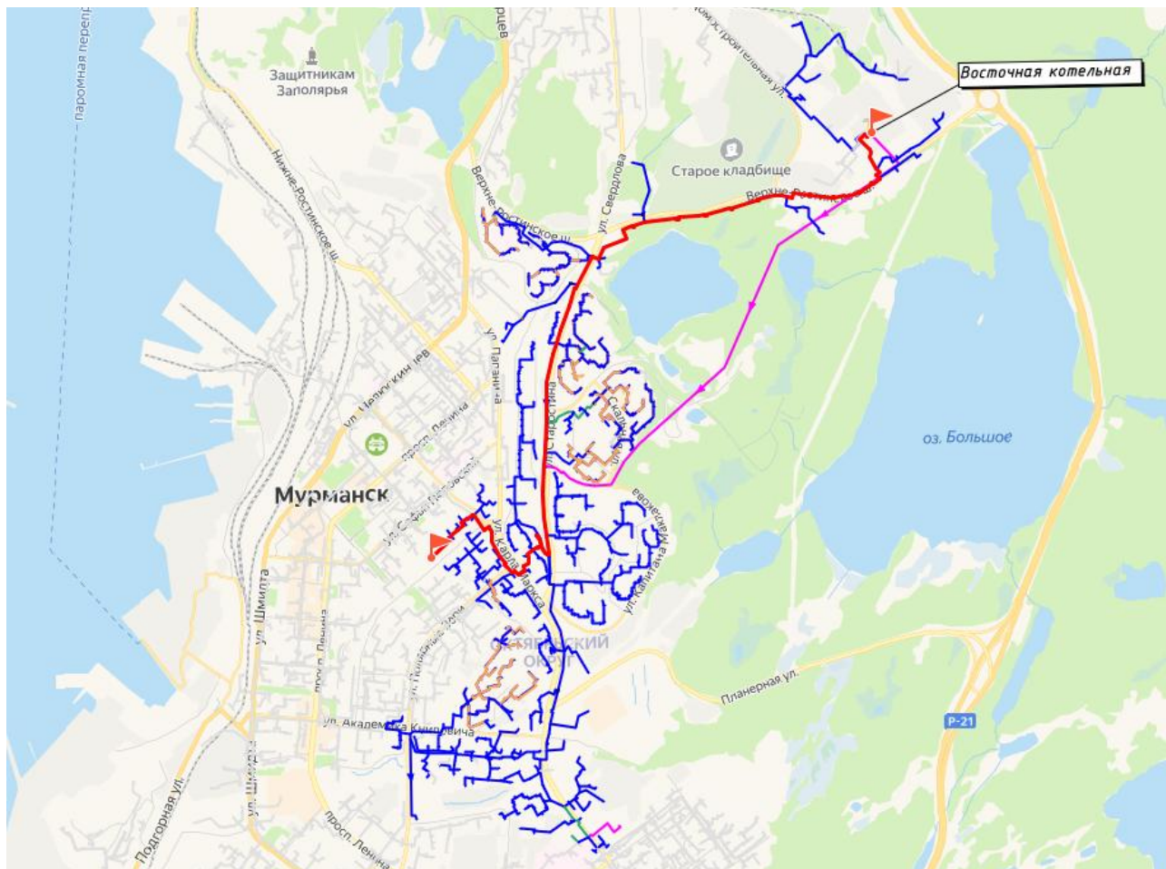
Рисунок 4.11 Путь для построения пьезометрического графика от Восточной котельной до перспективного потребителя Храм на Буркова
