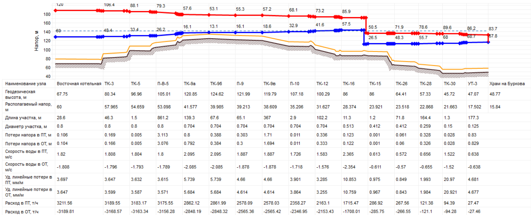
Рисунок 4.12 Пьезометрический график участка тепловой сети от Восточной котельной до перспективного потребителя Храм на Буркова
