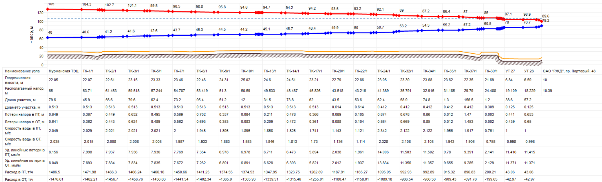
Рисунок 4.6 Пьезометрический график участка тепловой сети от Мурманской ТЭС до ОАО «РЖД» (Портовый, 48)
