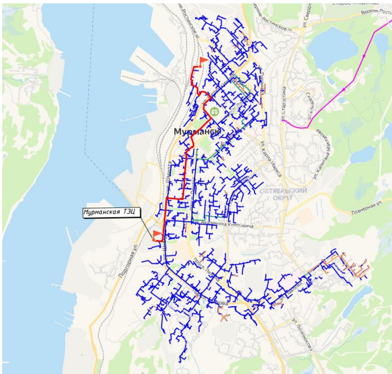
Рисунок 4.5 Путь для построения пьезометрического графика от Мурманской ТЭЦ до ОАО «РЖД» (Портовый, 48)
