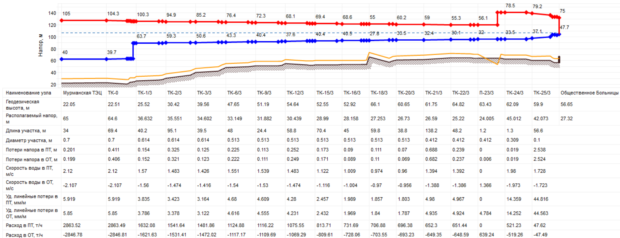
Рисунок 4.8 Пьезометрический график участка тепловой сети от Мурманской ТЭС до потребителя ул.Павлова, д.6, корп.2
