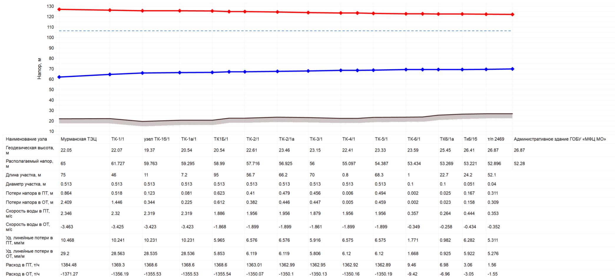
Рисунок 4.4 Пьезометрический график участка тепловой сети от Мурманской ТЭЦ до административного здания
