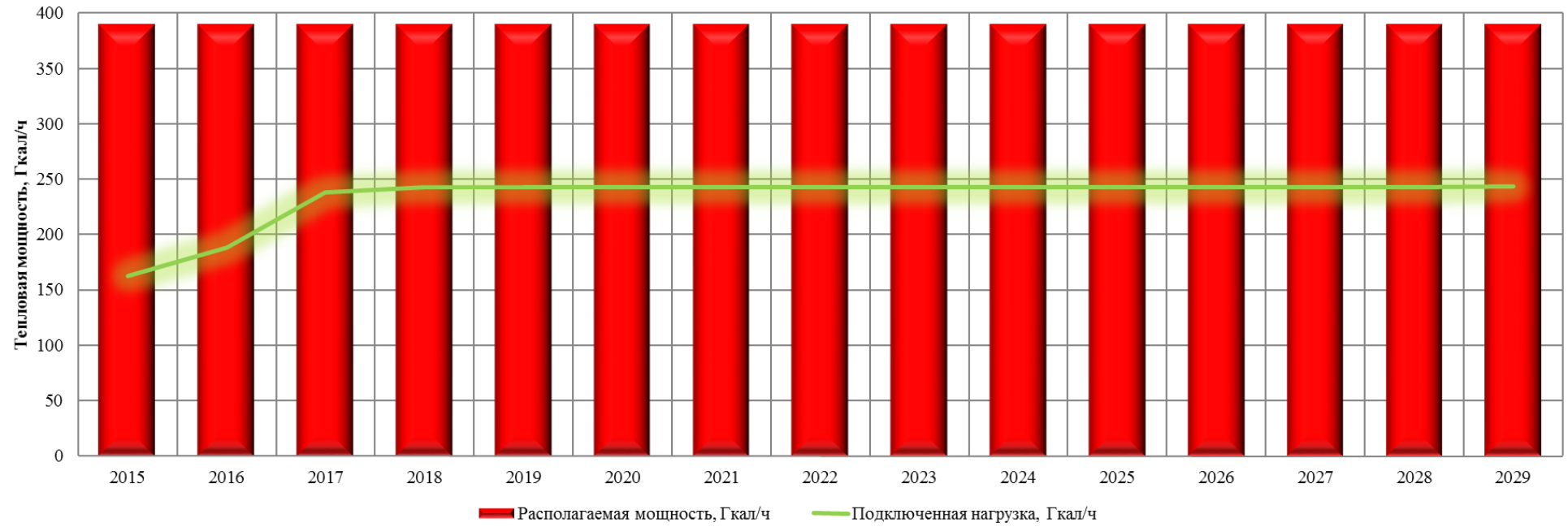
Рисунок 6.11 - Баланс тепловой мощности котельной Восточная для Сценария 1
