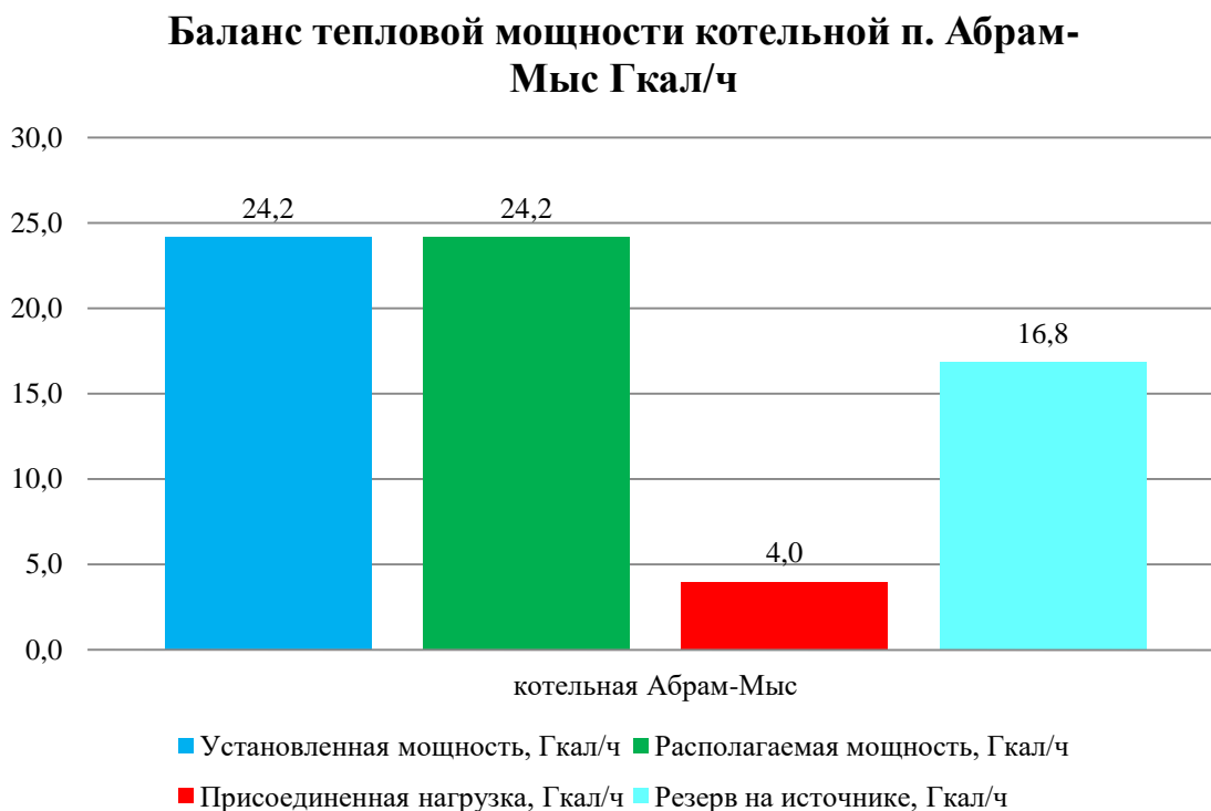
Рисунок 6.19 - Баланс тепловой мощности котельной п. Абрам-Мыс
