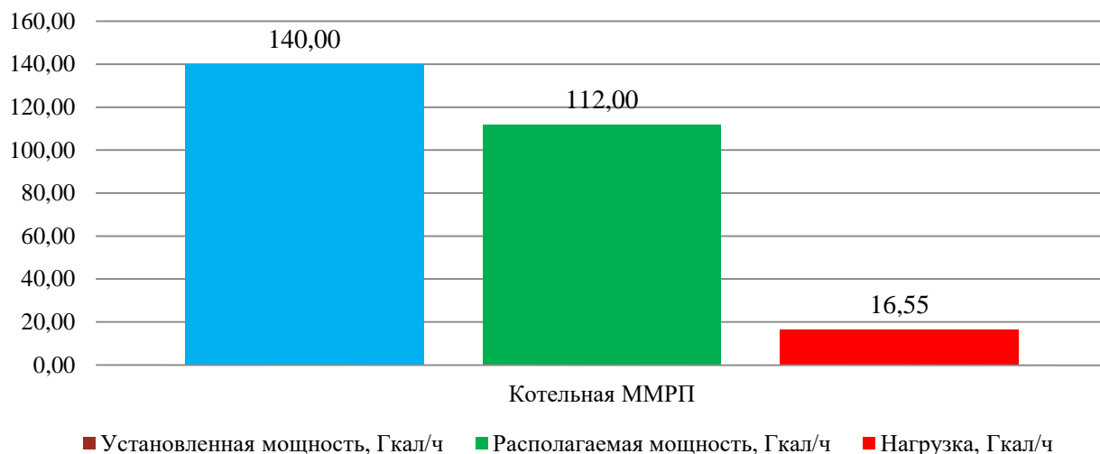
Рисунок 6.20 - Баланс тепловой мощности котельной
