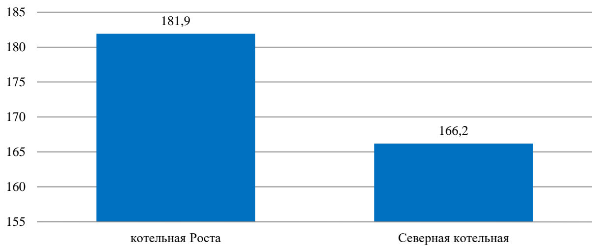
Рисунок 6.15 - Удельные расходы топлива на Северной котельной и котельной Роста
