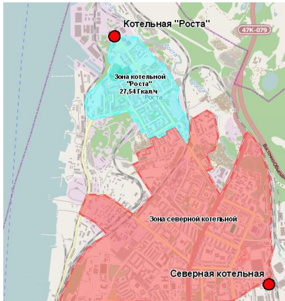
Рисунок 6.14 - Зоны теплоснабжения котельной Роста и Северной котельной
