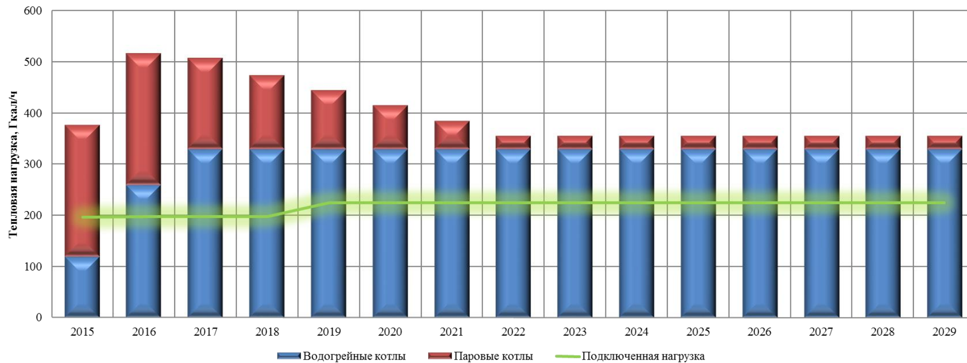
Рисунок 6.13 - Баланс мощности и нагрузки котельной Северная по 2 сценарию
