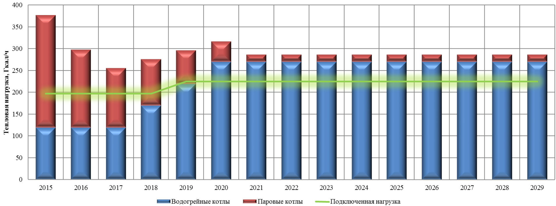
Рисунок 6.12 - Баланс мощности и нагрузки котельной Северная по 1 сценарию
