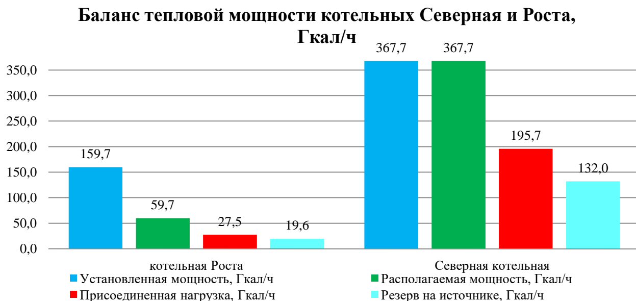
Рисунок 6.16 - Баланс тепловой мощности котельных Северная и Роста
