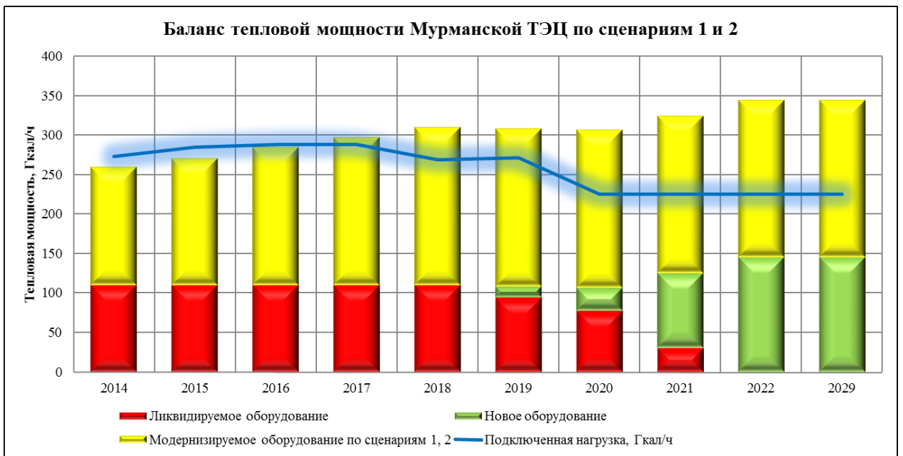
Рисунок 6.10 - Баланс тепловой мощности МТЭЦ на период актуализации схемы теплоснабжения
