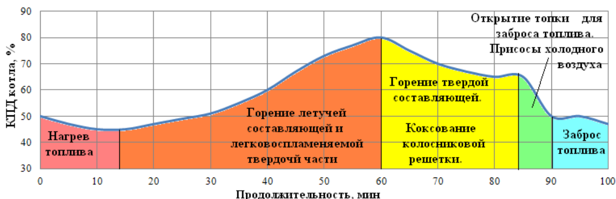
Рисунок 6.18 - Циклическая зависимость КПД котла с ручной подачей топлива
